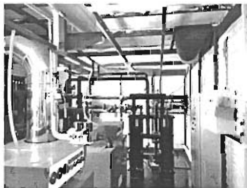
Оборудование блочно-модульной котельной в Свияжском сельском поселении
